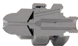
内部混合，压力装置： 扇形喷雾
